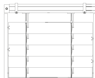
Boční vedení v lištách
